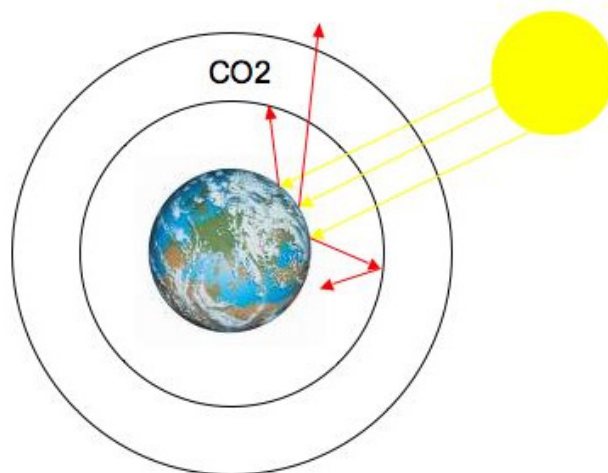
Figuur 2.1 Broeikaseffect
