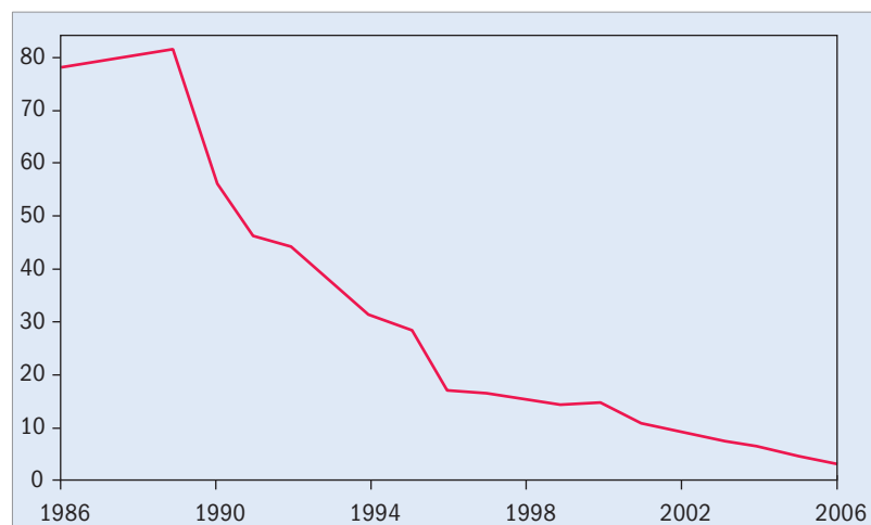
FIGUUR 1.4 Het wereldwijde gebruik van CFK's in de jaren 1986 tot 2006. De eenheid of de verticale as is 'ODP Metric Tonnes' (maal 10^4 ). ODP staat voor 'Ozone Depleting Power', het vermogen om ozon af te breken
